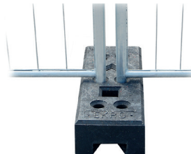
105681 Kunststoffsockel für Mobilzaun Gewicht: 25kg
