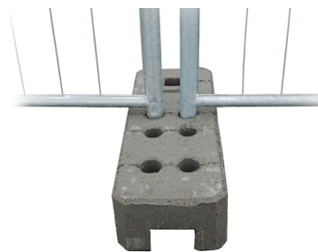
Betonsockel für Mobilzaun Gewicht: 33kg ARTNR. 105679
