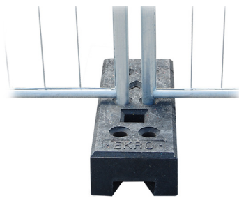
Kunststoffsockel für Mobilzaun Gewicht: 25kg ARTNR. 105681
