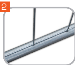
2 Gitter mittig im Rahmen verschweißt
