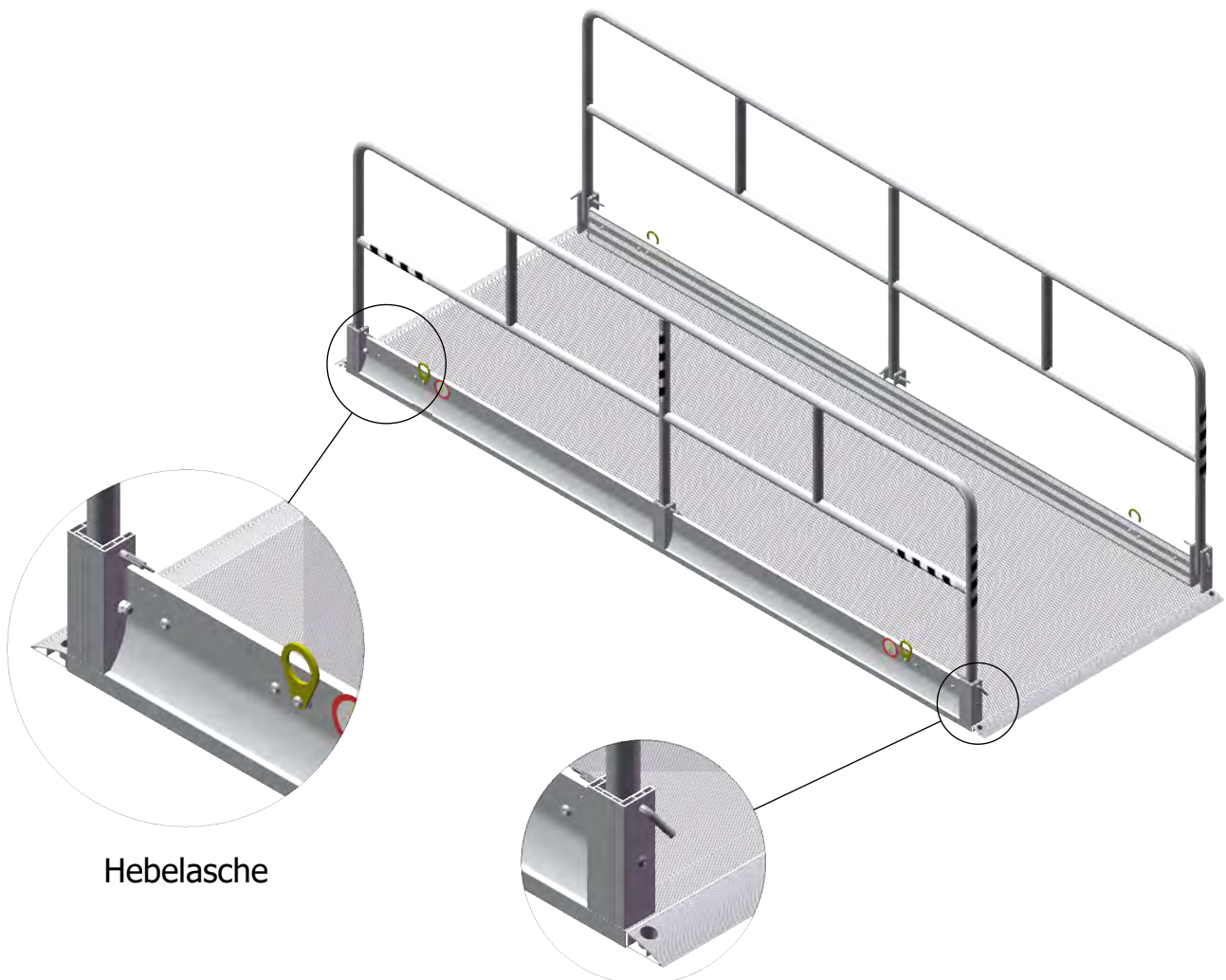
Befestigungspunkte
