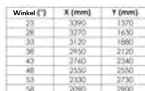
205759 Bautreppe Alu 70 (18 Stufen)
