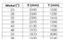
205760 Bautreppe Alu 70 (15 Stufen)
