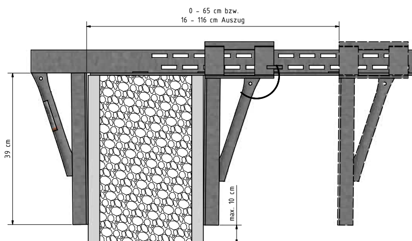
Anwendung Schalungswinge
