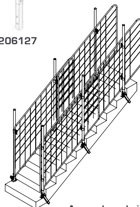
Anwendungsbeispiel EP Treppenschutzgitter 220/140
