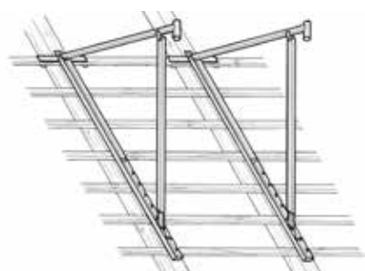
Anwendung Dachabstellkonsole
