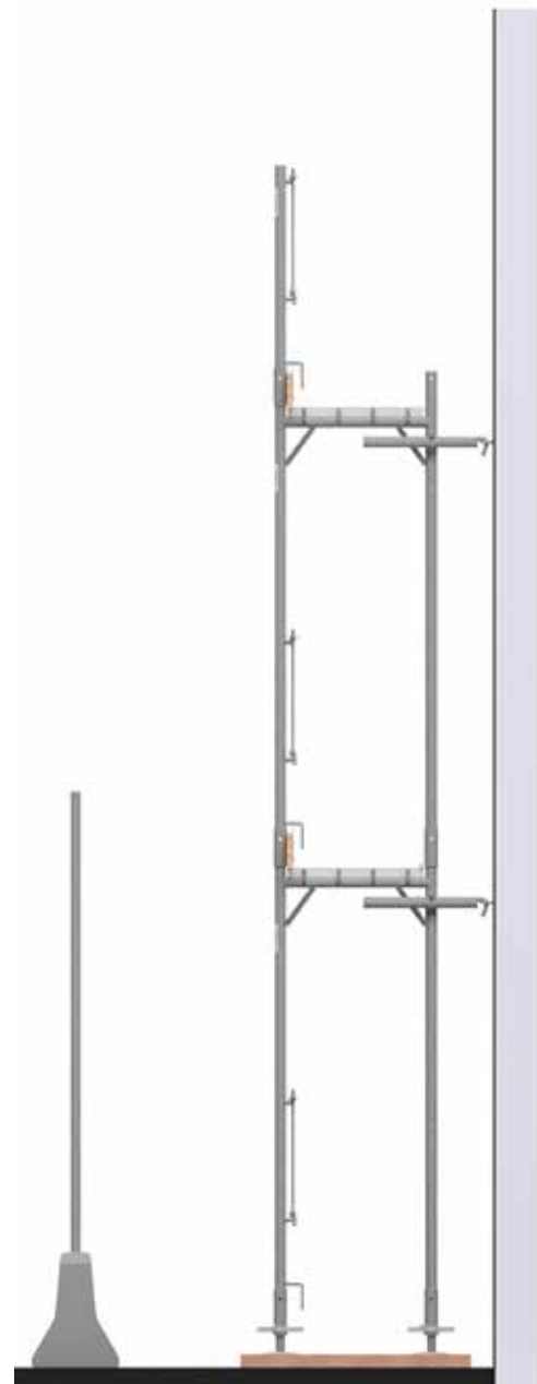
Anfahrerschutz z.B. mit CITYBLOC®, Mobilzaunadapter und Mobilzaun
