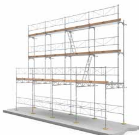
Durchgangsbreite -P 1,8m
