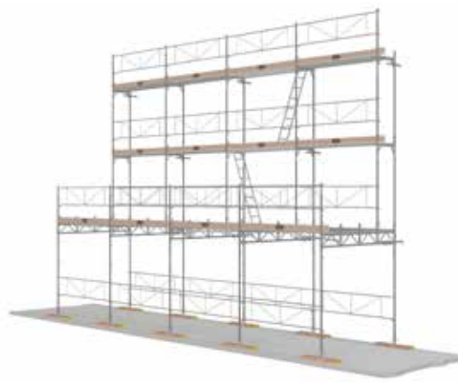
Durchgangsbreite -P 2,5m
