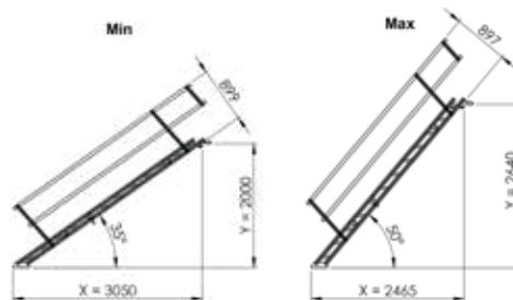
205761 Bautreppe Alu 70 (12 Stufen)
