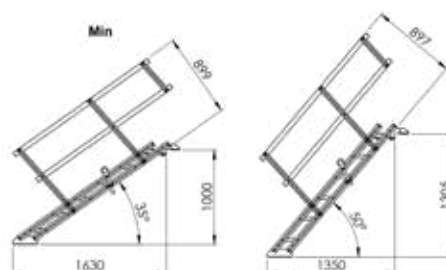
205763 Bautreppe Alu 70 (6 Stufen)
